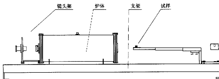
图 1 熔化温度测试装置
